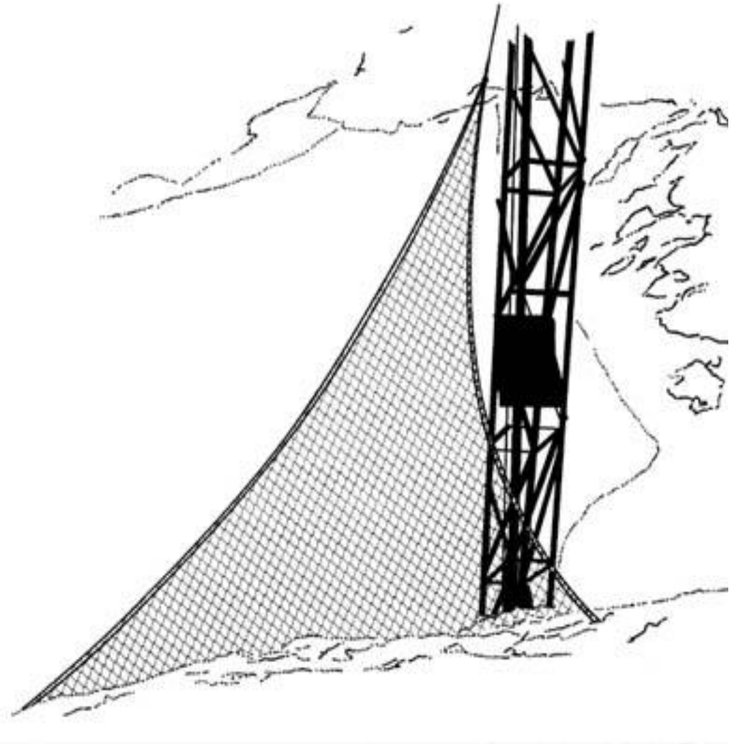
Trikotna mreža, ki se običajno namešča pred stebre žičniških naprav
